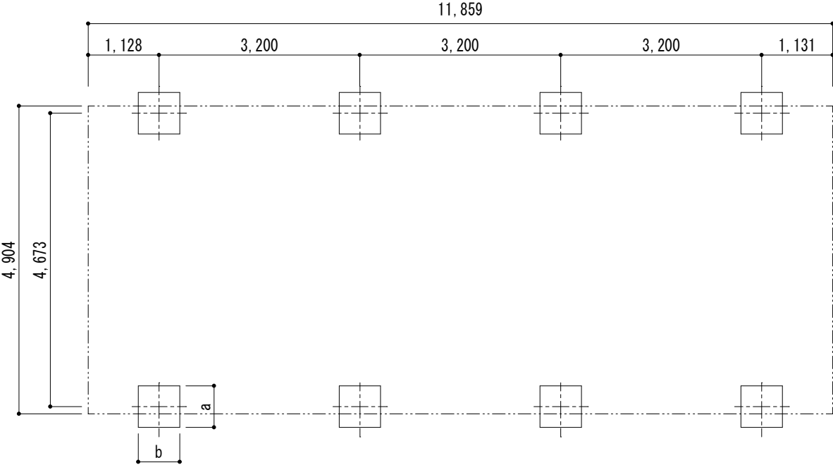
■基礎配置図
